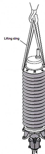
Рис. 3. Подъём КМ стропами, закреплёнными под верхним фланцем композитного изолятора
